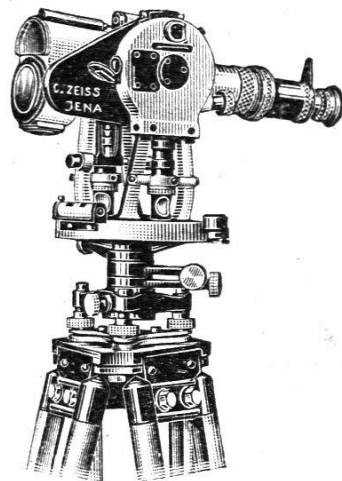
Reduktions-Tachymeter
