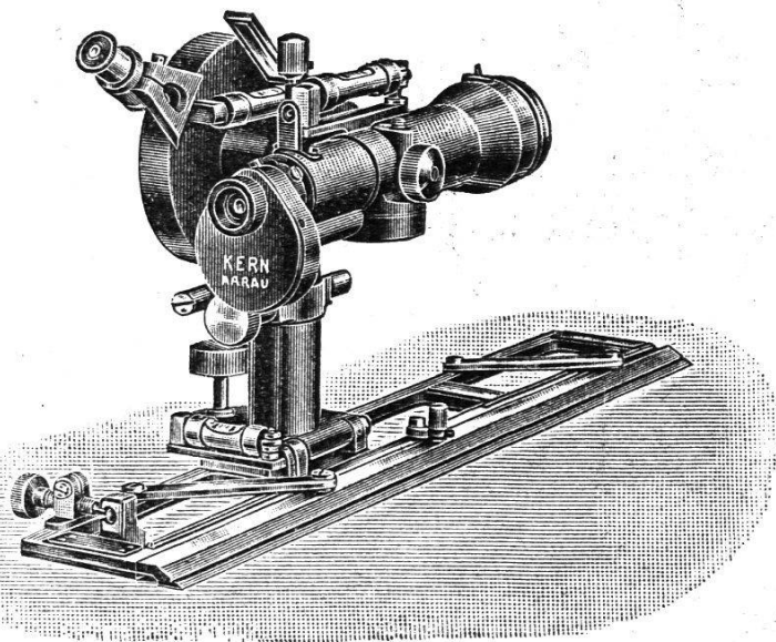
Kippregel Nr. 79
