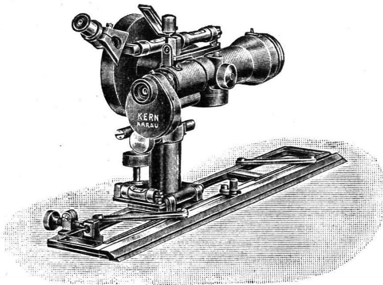
Kippregel Nr. 79
