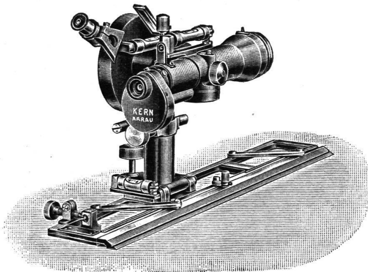
Kippregel Nr. 79
