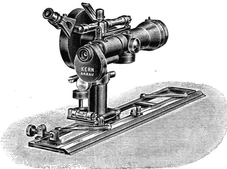
Kippregel Nr. 79
