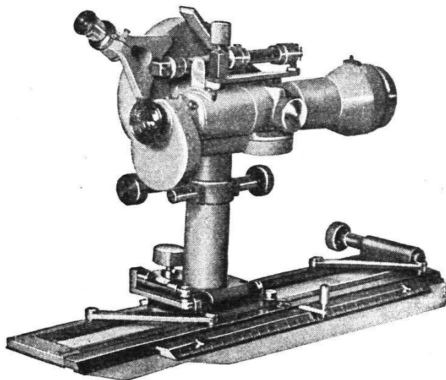
Kippregel Nr. 79
