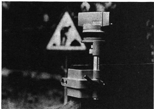
Klemmstativ GST 7
