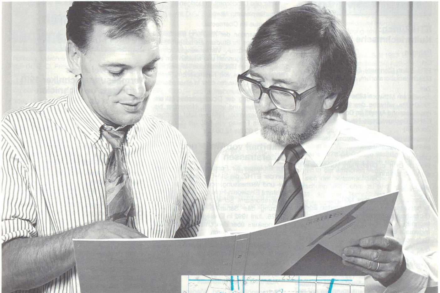
* Geografisches Informations-System
