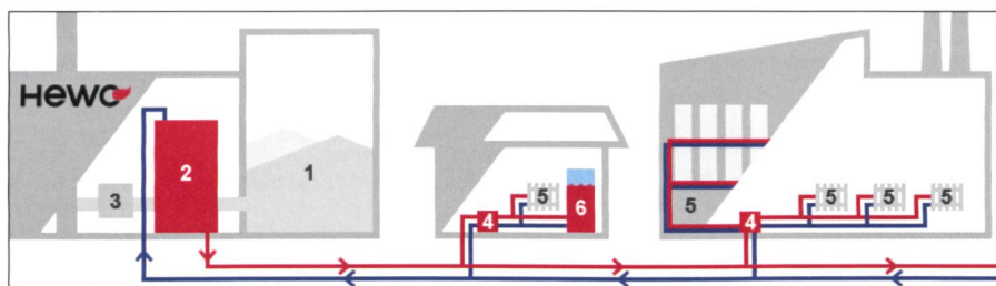
Abb. 1: Wärmekreislauf 2 .
