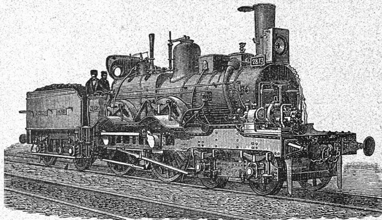
Schnellzugs-Lokomotive.
