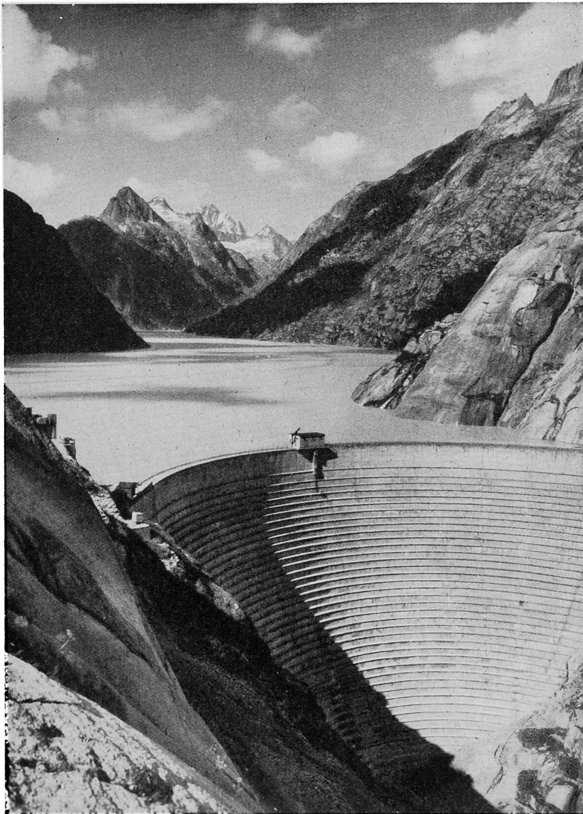
Der Grimselsee mit der 114 m hohen Spitaldammsperre. Im Hintergrund Finsteraarhorn (4274 m); rechts davon, über dem Tierberggletscher mit Escherhorn (3100 m), das Agassizhorn (3953 m); links (schwarz) der Vorder-Zinggenstock (2920 m)
