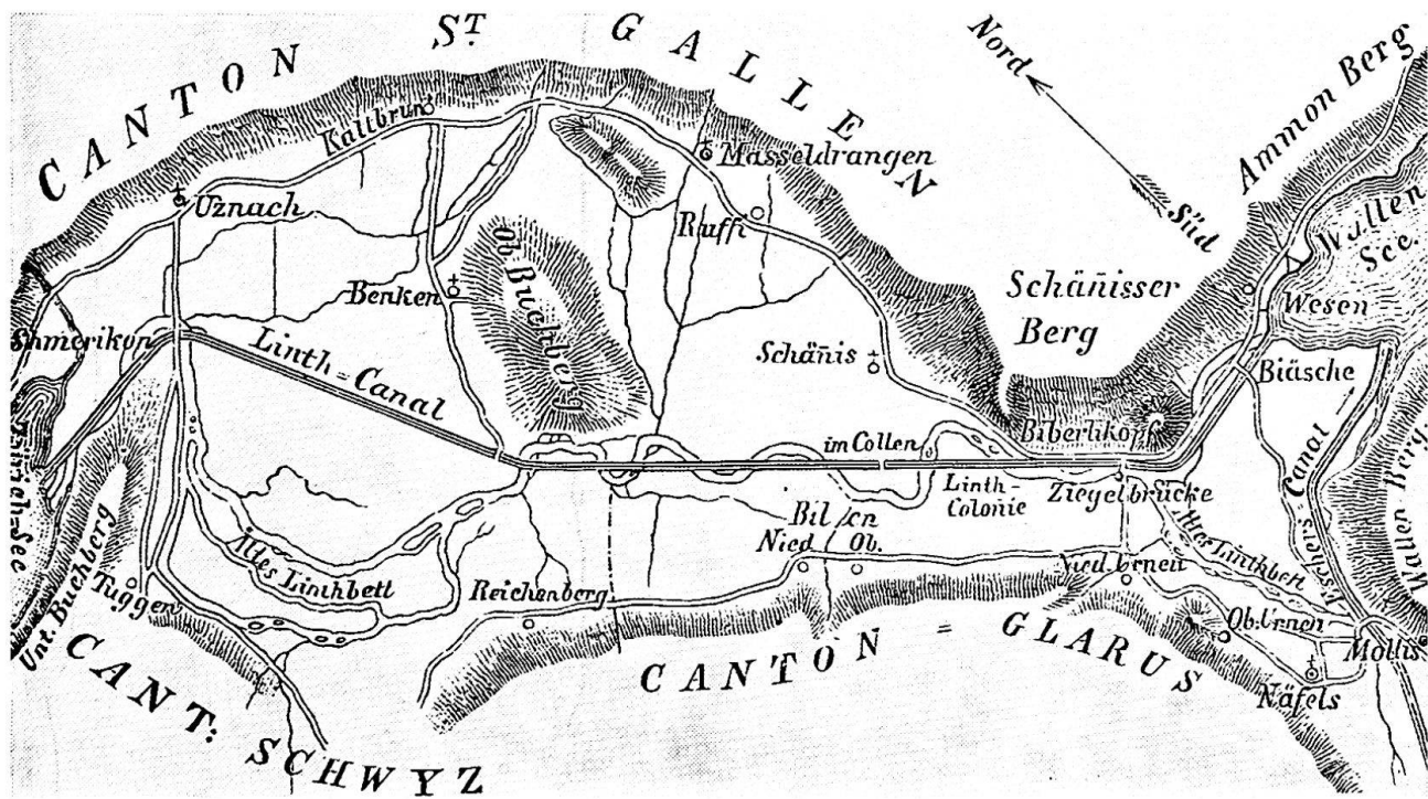
Abb. 2 Der alte Linthlauf und das unter der Leitung Eschers durchgeführte Korrekptionswerk.
