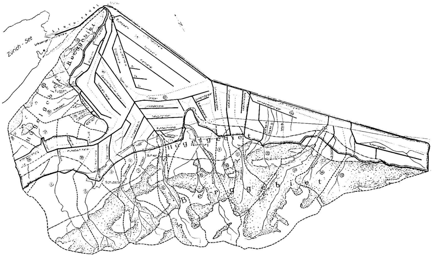
Abb. 5 Plan der modernen Gewässerkorrektur der linksseitigen Linthebene. Aus dem Schlußbericht der Melioration der Linthebene, 1966.
