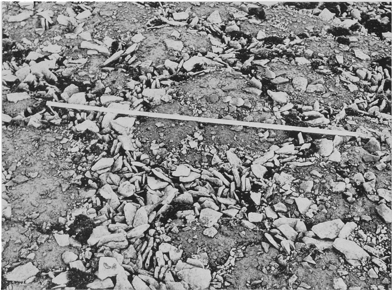
Abbildung 2. Steinpolygone, ein Steinnetz bildend (Sverdruphamaren). Dunkle Flecken: Vegetation, Maßstab 120 cm. Die von den Steinpolygonen umgrenzte Feinerdefläche ist von feinen, «sekundären» Steinpolygonen gemustert
