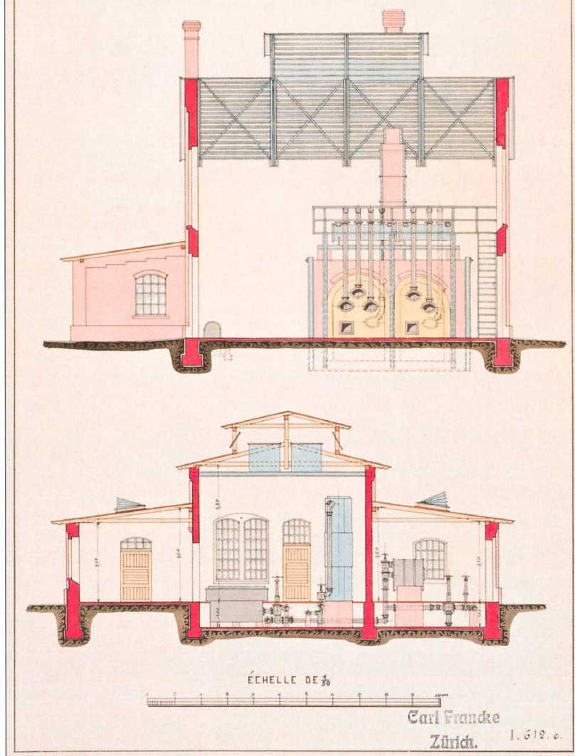
Détail d'un projet d'usine à gaz à Bulle de la maison Carl Francke à Zurich. 70 x 44 cm, encre et aquarelle. AVB. © Musée gruérien. Photo Primula Bosshard
