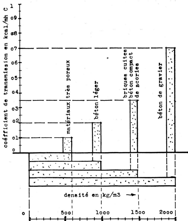
Fig. 2. Rapport entre le coefficient de transmission calorifique et la densité des matériaux de construction.
