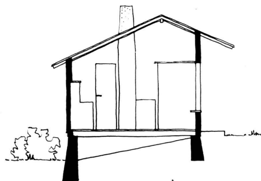
Coupe.
