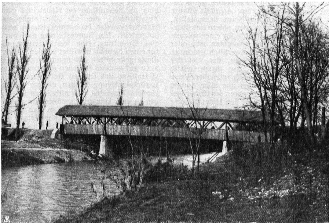
Abb. 21. Die neue Birsebrücke bei Münchenstein. Ein Werk schweizerischer Genietruppen. Die photographischen Aufnahmen stammen von Kuratle, jene der Masken von Ph. und E. Link, beide in Zürich. Fig. 21. Le nouveau pont de la Birse à Münchenstein, exécuté par les troupes suisses du génie.
