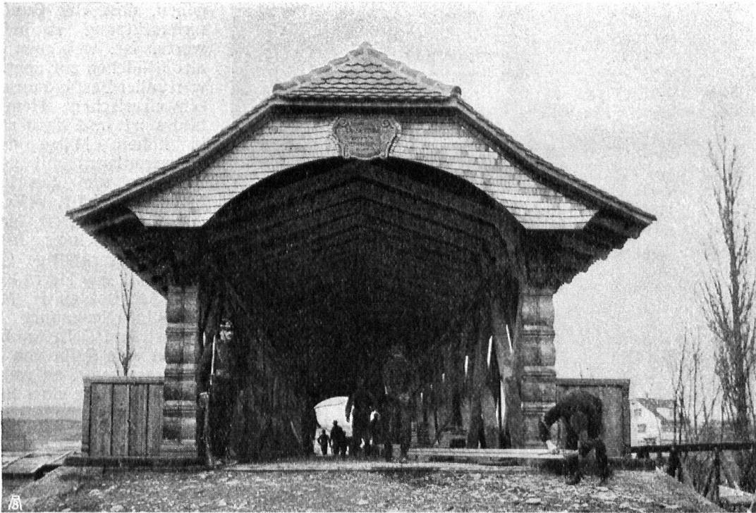
Abb. 20. Brückenkopf der hölzernen Birsebrücke in Münchenstein. Mit Holzschnitzerei, Schindelvorschirm und Ziegeleindeckung. — Fig. 20. Tête du pont de Münchenstein. Sculptures en bois. Toiture de tuiles. Parois protectrices en clavins.
