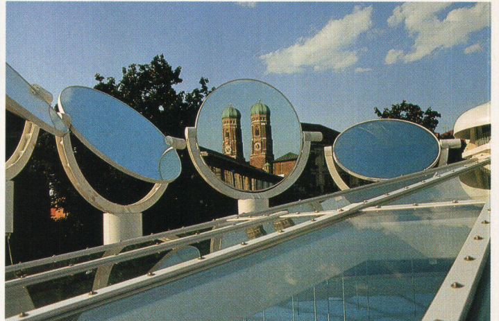
Mit Heliostaten kommt Tageslicht in Innenräume z. B. bei BMW in München
