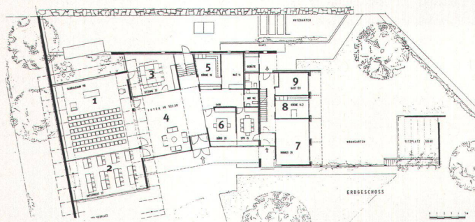
Grundriss Erdgeschoss
