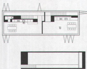
Grundriss EG
