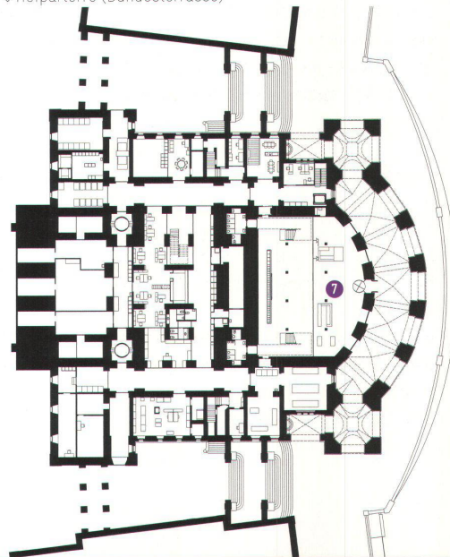
∨ Tiefparterre (Bundesterrasse)
