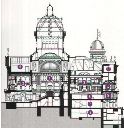
^ Querschnitt
