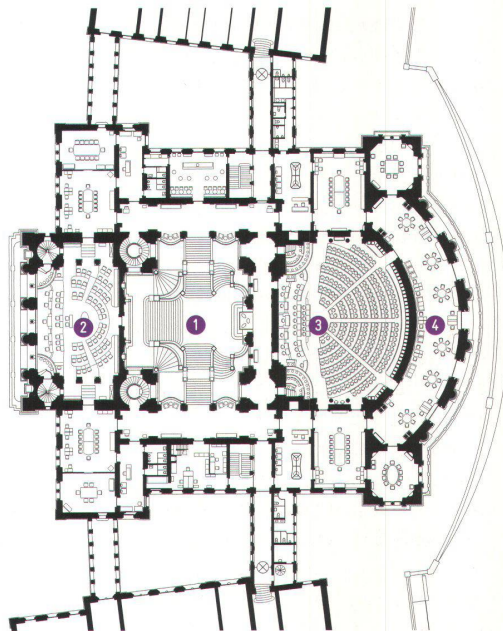
^ 1. Obergeschoss (Hauptgeschoss)
