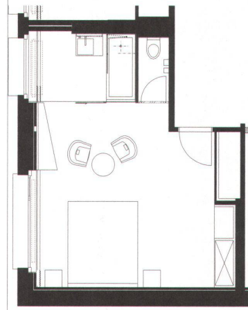
▽ Grundriss Doppelzimmer Superior, 36 m 2
