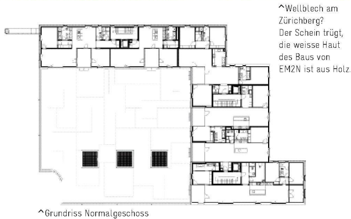
^Grundriss Normalgeschoss
