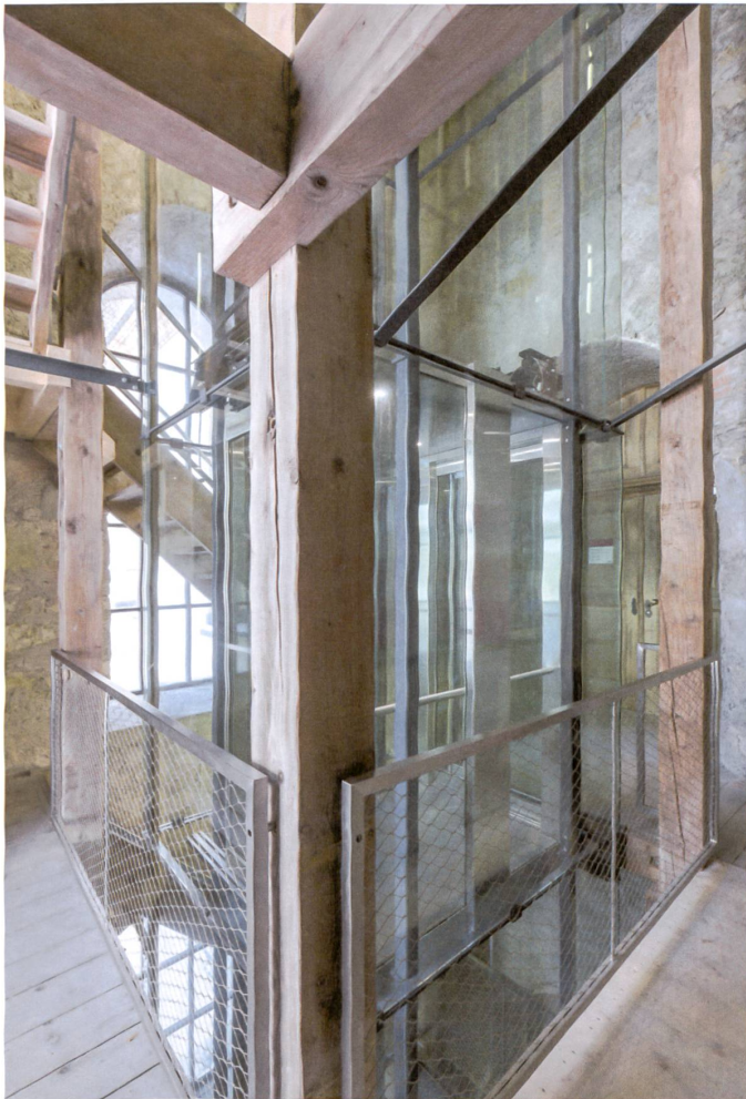
Mit grösstmöglicher Transparenz wollte der Architekt den Lift ins Auge der Holzterrasse einfügen.
