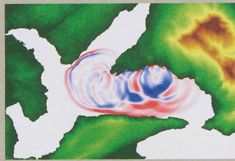
Des vagues de 3 mètres se propagent une minute après le glissement de terrain de Weggis en 1601.
