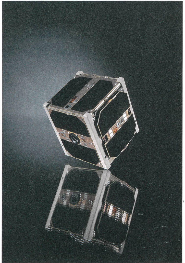
Nur balancieren kann er nicht: Der Studierenden-Satellit weist eine Kantenlänge von zehn Zentimetern auf und wiegt 820 Gramm. Bild: Alain Herzog/EPFL
