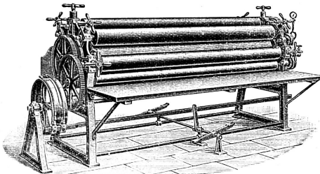
Dampf-mangel-Trocken- und Plättmaschine für glatte Wäsche in 4 verschiedenen Längen, mit Heizcylinder von 500 mm Durchmesser, 4 Andruck- u. 1 Abgewalze, mit höchster Leistung u. Vollkommenheit.
