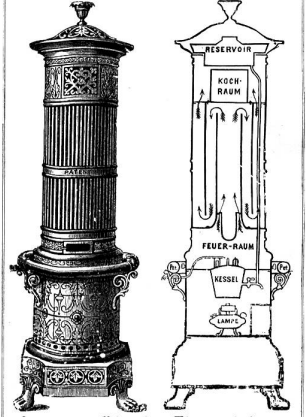
Petroleum-Ofen für Zimmerheizung von Robert Schulz.
