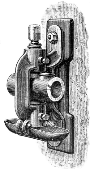
Geschlossenes Wandlager
