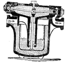
Condensationstöpfe
