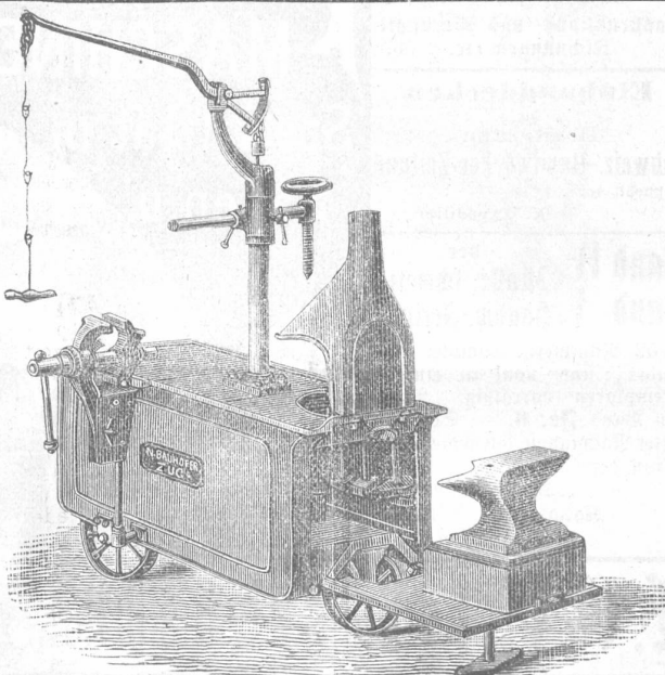
Montir-Schmiede (dieselbe erlitt nach Abbildung mehrfache Aenderungen). Bequem fahrbar, mit Ambos, Schraubstock und Bohrmaschine, grossem verschliessbarem Werkzeugschrank; in 3 Grössen.
