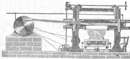
Horizontal-Sägegatter.
