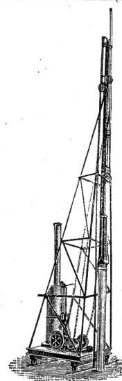
Rammarbeiten. Besteingerichtete Gerüste auf Dielenunterlagen, Geleisen und Pontons. [380 (M 10226 Z)]
