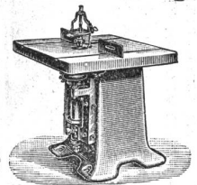
Fräs-Maschine.
