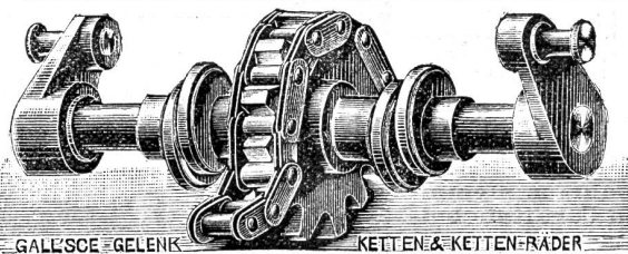
GALL'SCHE GELENK
