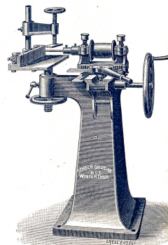
Langlochbohrmaschinen mit und ohne Stemmaparat.
