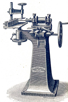
Langlochbohrmaschinen mit und ohne Stemmaparat.
