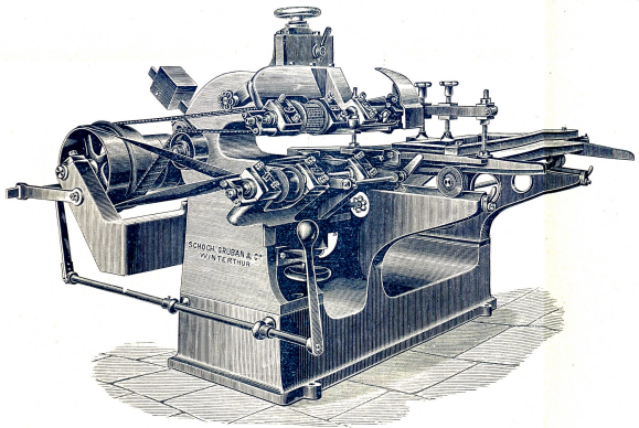
Zapfenschneid-Maschinen.
