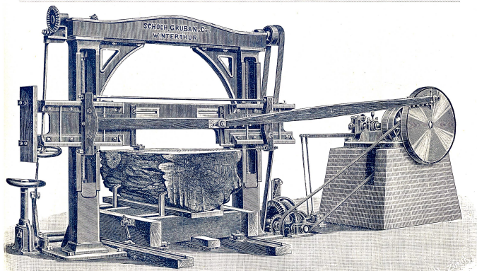
Patent-Horizontalgatter mit einem Vorschub bis zu drei Meter per Minute. Patent Doppelsägerahmen. Scieries horizontales brevetées. Aménage jusqu'à trois mètres par minute. Châssis breveté pour deux lames.
