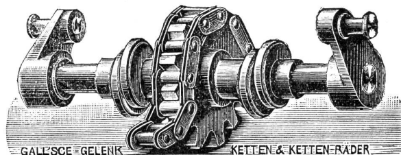
GALLSCHE GELENK KETTEN- & KETTEN-RÄDER
