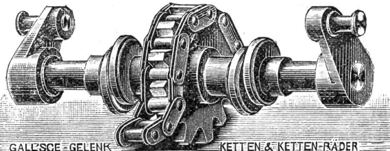
GALLSCHE GELENK KETTEN- & KETTEN-RÄDER
