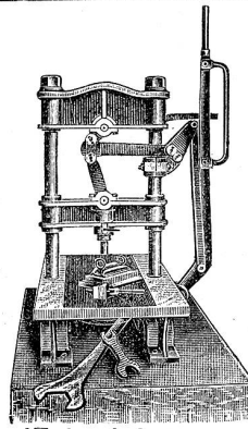
Knishebelpresse
