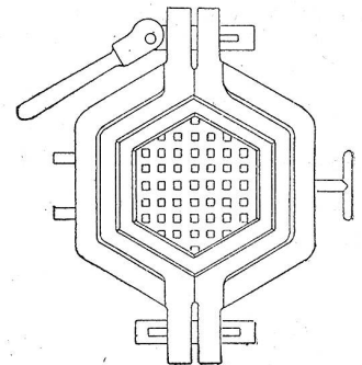
Sechseck-Form
