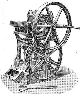
Excenterpresse
