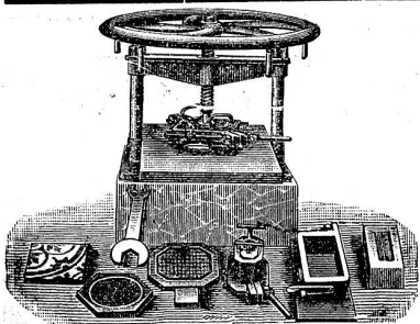
Spindelpresse
