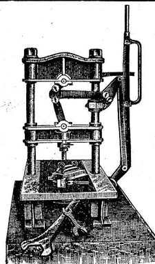
Kniehebelpresse
