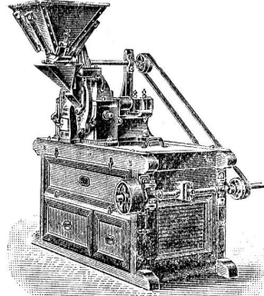
Universalmühle mit Siebvorrichtung.
