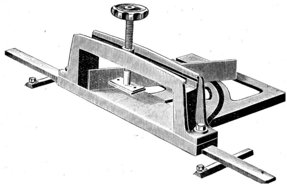
Zapfenschneidtischchen
