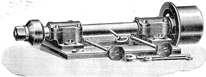
Kreissägenwelle
