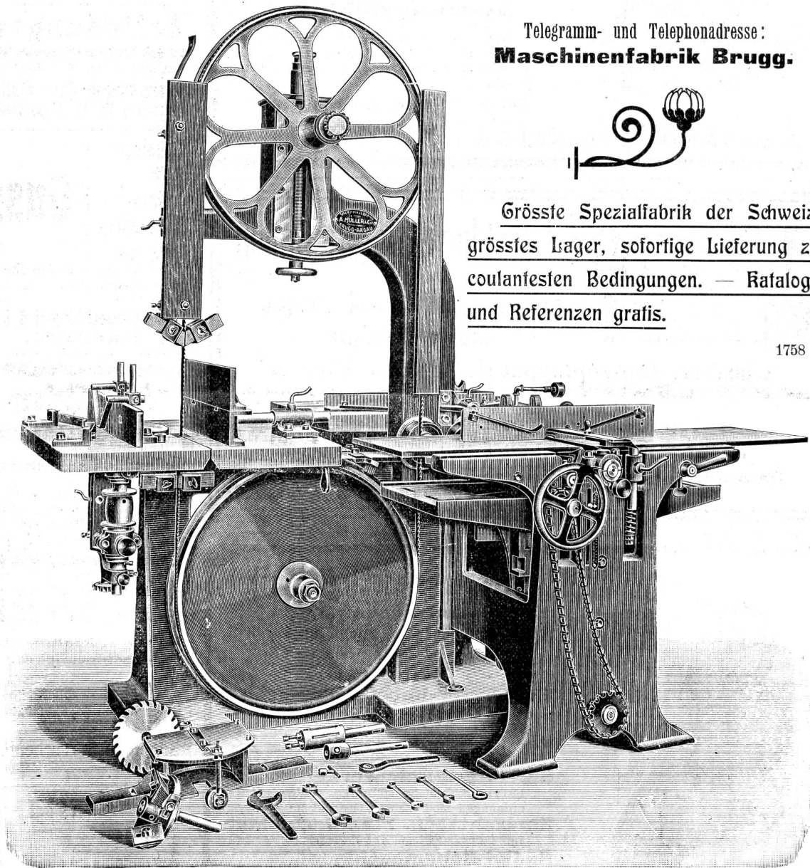
Universalsmaschine No. 3.
