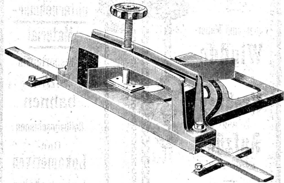
Zapfenschneidtischchen
