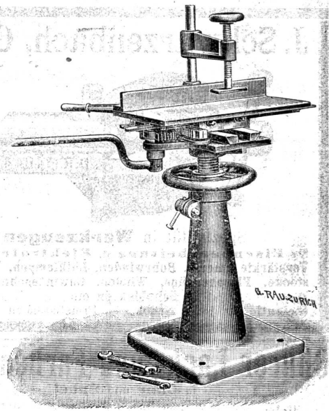
Bohrständer
