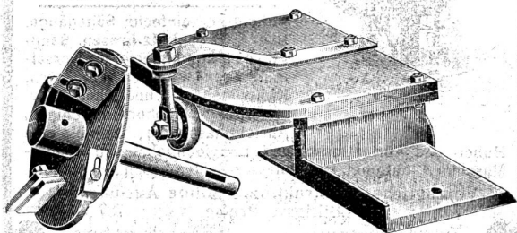
Abplattkopf mit Schutzvorrichtung
