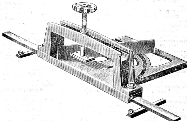
Zapfenschneidmaschine
