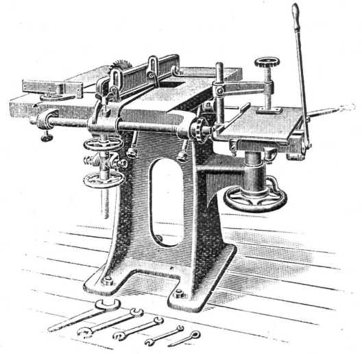
Kreissäge kombiniert mit Langlochbohrmaschine.
