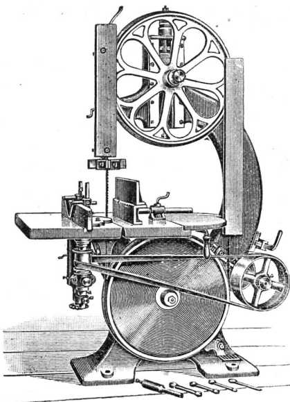
Bandsäge kombiniert mit Kehlmaschine.
