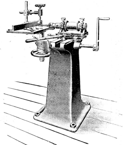
Langlochbohrmaschine.
