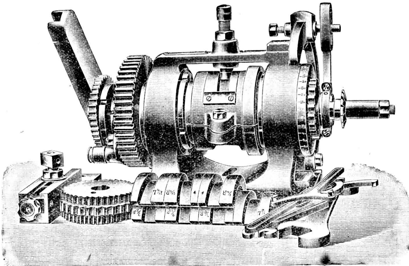
Hinterdreh-Apparat No. 1.
