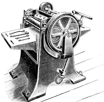
Dickehobelmaschine.
