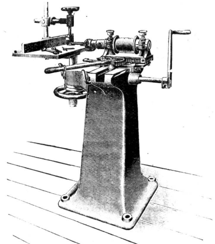
Langlochbohrmaschine.
