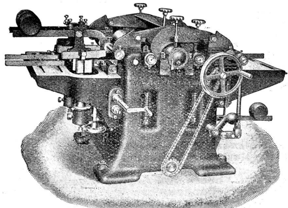
Dreiseitige Hobelmaschine.
